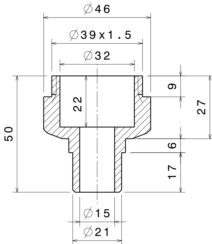
Coupe A-A
